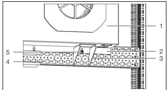
Imagen 4: Disposición de la unidad interior
