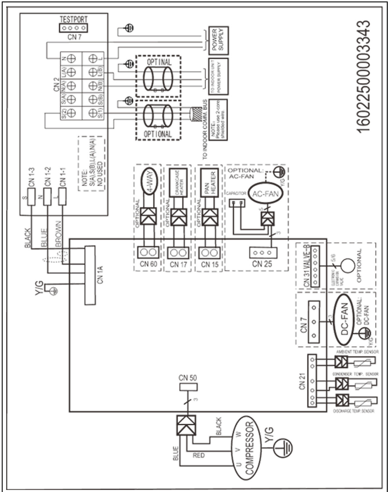
Imagen 25: Diagrama de circuitos unidad exterior SK 3311.490 y SK 3311.491
