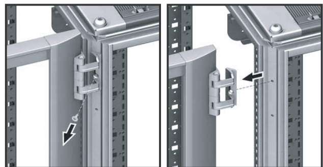
Fig. 13: Removing a door hinge
